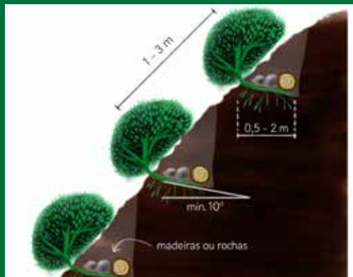
Figura 45: Desenho esquemático da técnica de banquetas.
