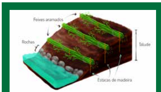
Figura 44: Desenho esquemático da técnica de feixes. (Adaptado de Li; Eddleman, 2002)
