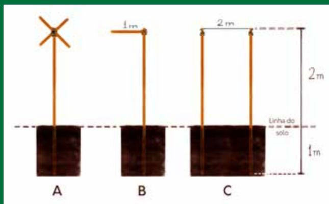
Figura 53: Ilustração da estrutura de poleiro artificial.
